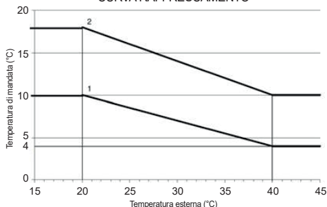
CURVA RAFFRESCAMENTO
